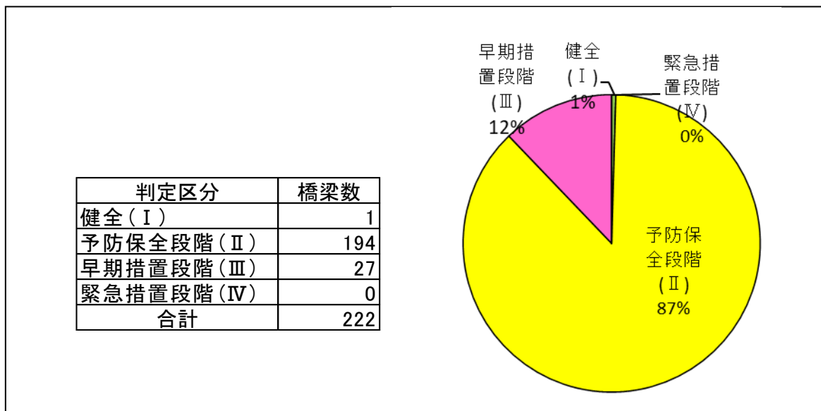
図 5 点検結果 (損傷区分毎の橋梁数) (令和 2 年 1 月末時点)
